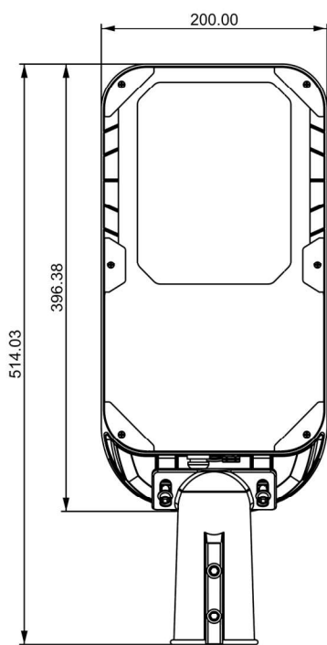
主视图
