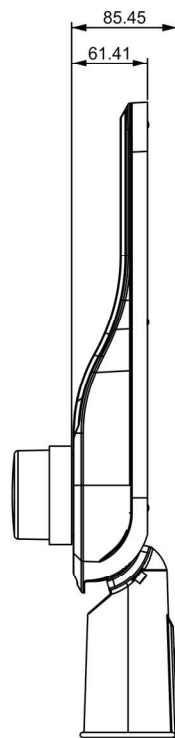
左视图
